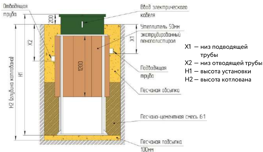
Рис. 1. Размеры станции ЕВРОБИОН АРТ
